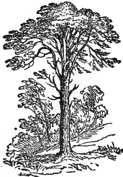
PINUS SYLVESTRIS. (Scotch Fir.)
